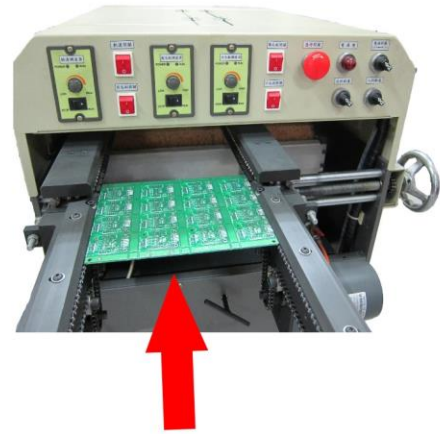
▲ PCB板入料方向
